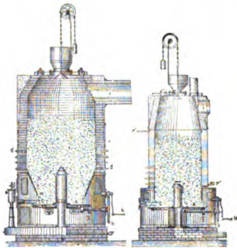
Taylorův generátor.
